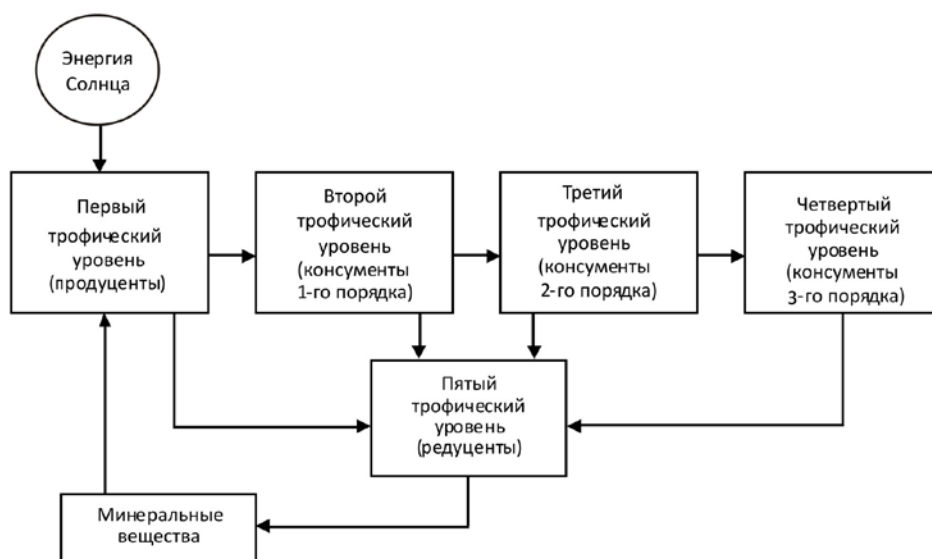
Рис. 7.1. Схема круговорота веществ и потоков энергии через пищевые цепи
