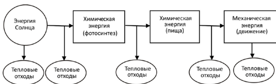
Рис. 7.2. Трансформация энергии в окружающей среде
